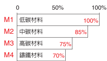
負載能力及鋼材之材質種類換算表
